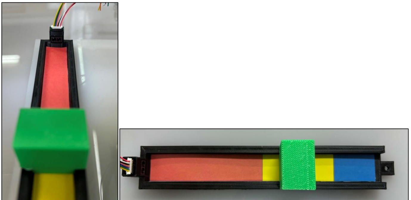
図7 測距用スライダ装置、スライダ、測距センサ設置図
