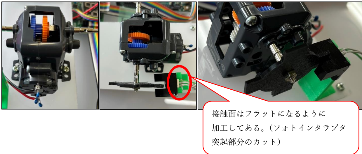
図6 DCモータとフォトインタラプタの設置図
