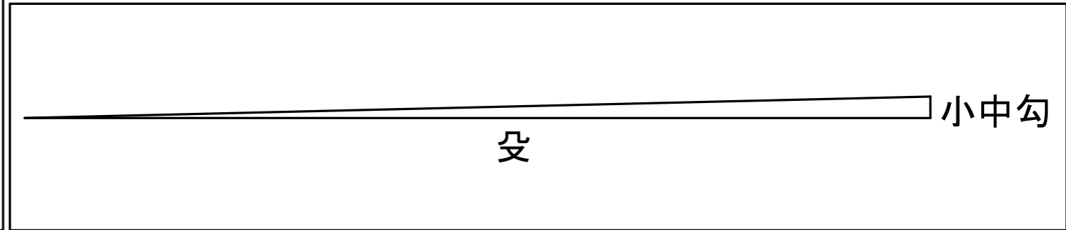
貫ほぞ孔上端・下端の勾配 (小中勾の返し勾配)
