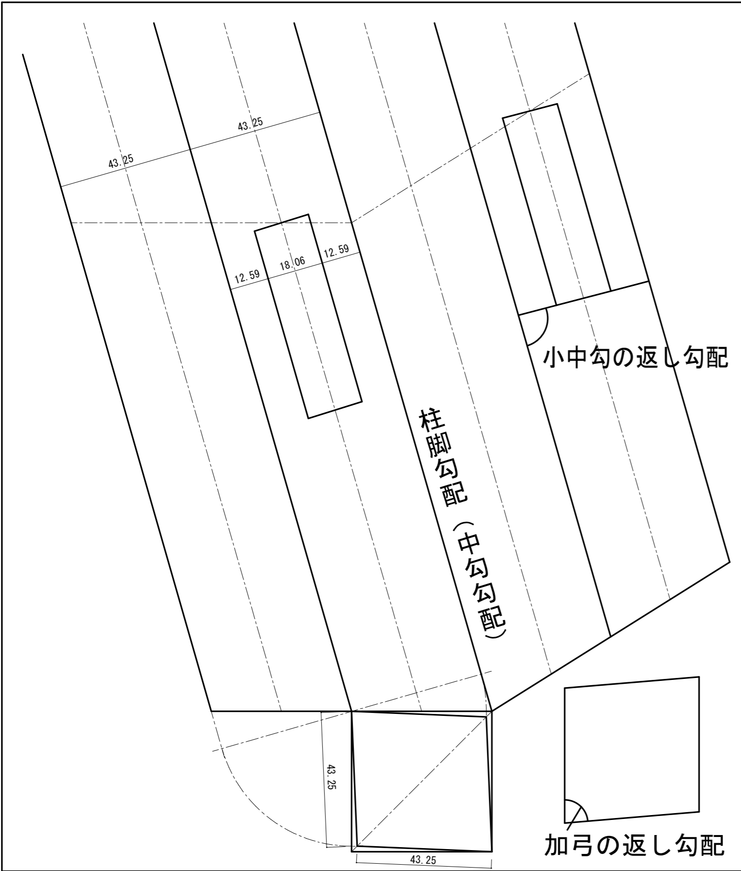
柱脚の癖 貫孔展開図
