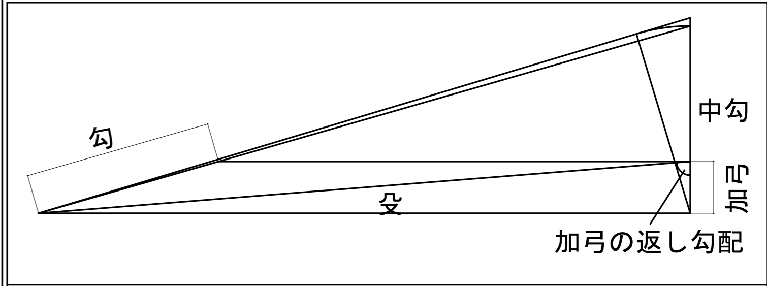
柱脚の癖 加弓勾配
